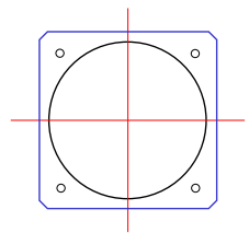
57mm Display (klassisch oder farbig) für alle LX-Systeme t = 140mm mit Stecker / with plug
