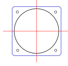
Zander ZS-1 Rundanzeige ZS-1 Vario indicator t = 70mm ohne Stecker / without plug Lautsprecher/Speaker T = 33mm
