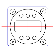
Filser Transponder TRT800 Funkgeräte / Radios ATR833 t = 250mm mit Stecker / with plug
