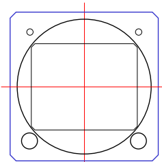
ILEC SN-10 Streckenrechner ILEC SN-10 Flight Computer t = 150 mm ohne Stecker / without plug
