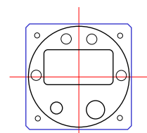
Dittel Funkgerät FSG90 / FSG2T t = ? (>150mm) ohne Stecker / without plug
