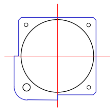
Winter: HM. mit D=57 t max. 110 mm
